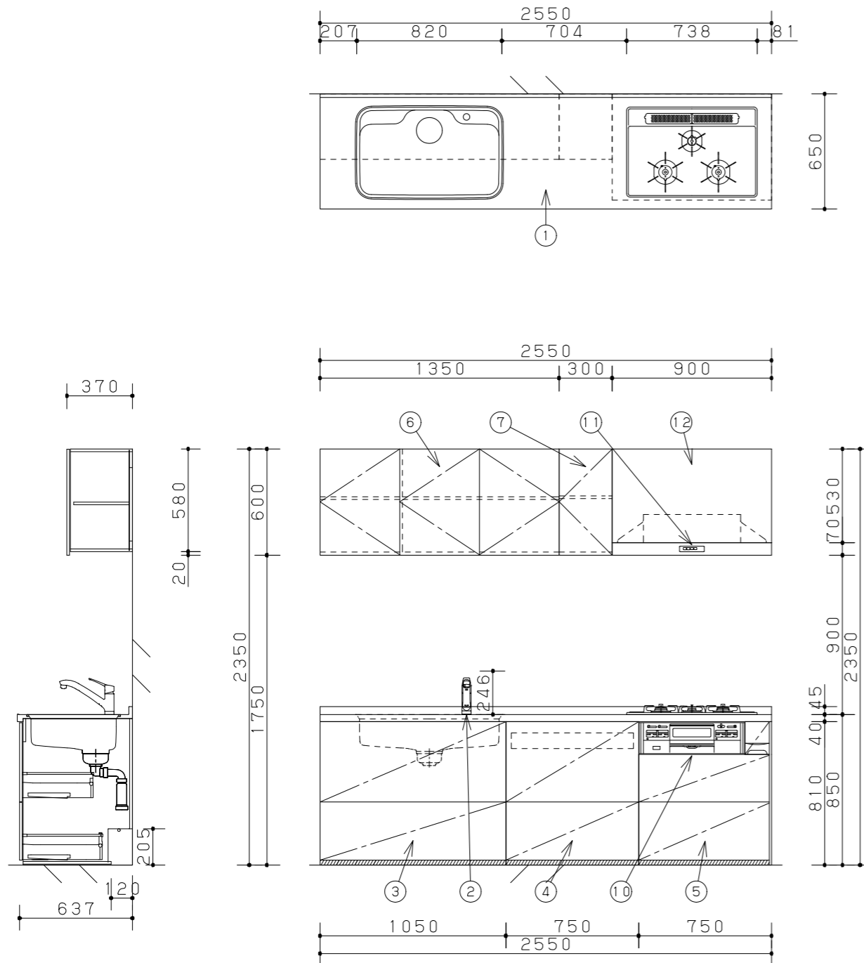
シンク断面
